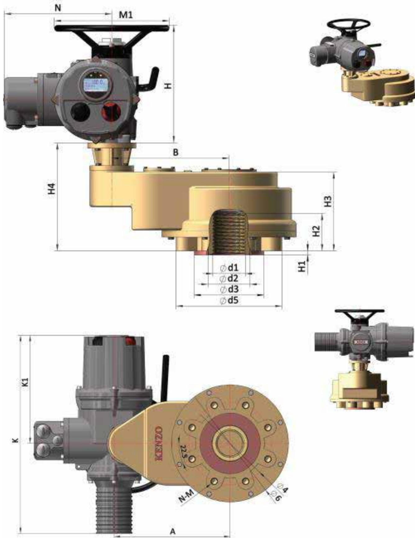
KZ/KZM +QST Габаритный чертеж
